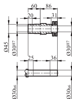
GFH/GFHZ/GFHF37输出轴
