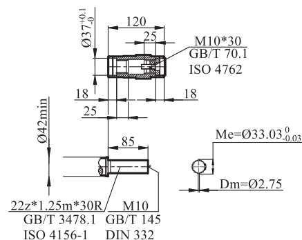
GFV/GFVZ/GFVF37输出轴
