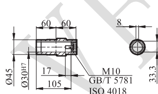
GFA/GFAZ/GFAF37输出轴
