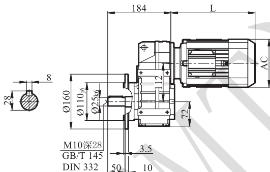
GFF37
