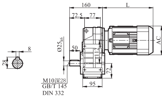
GF37
